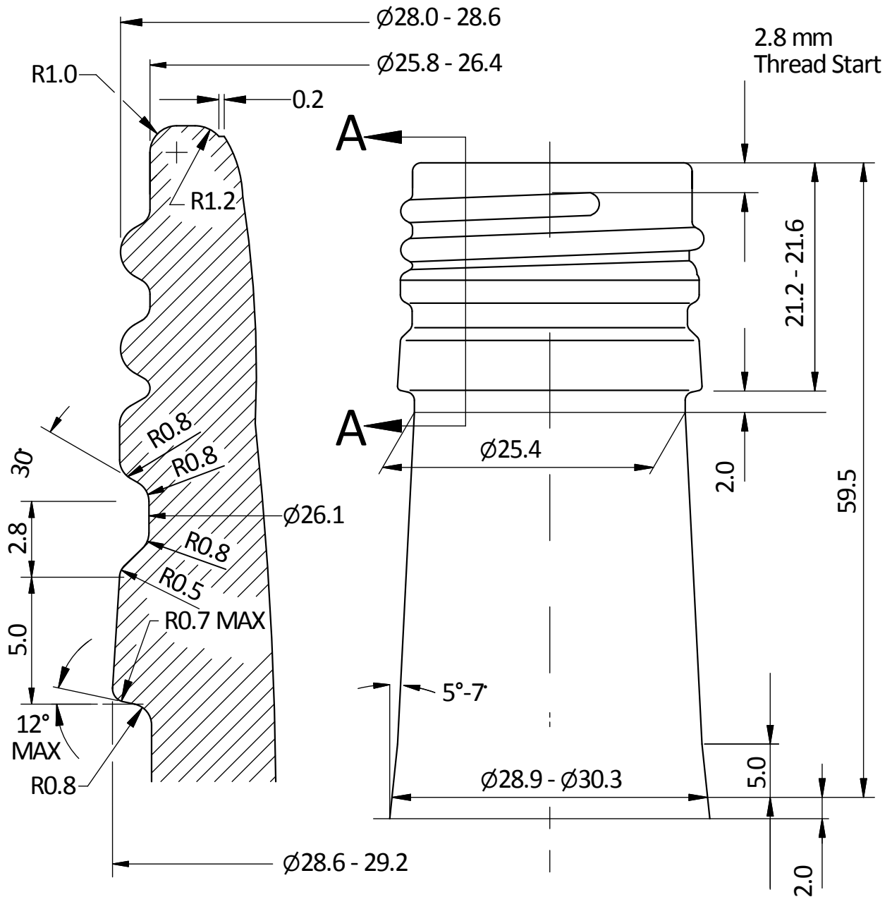
SECTION A-A
